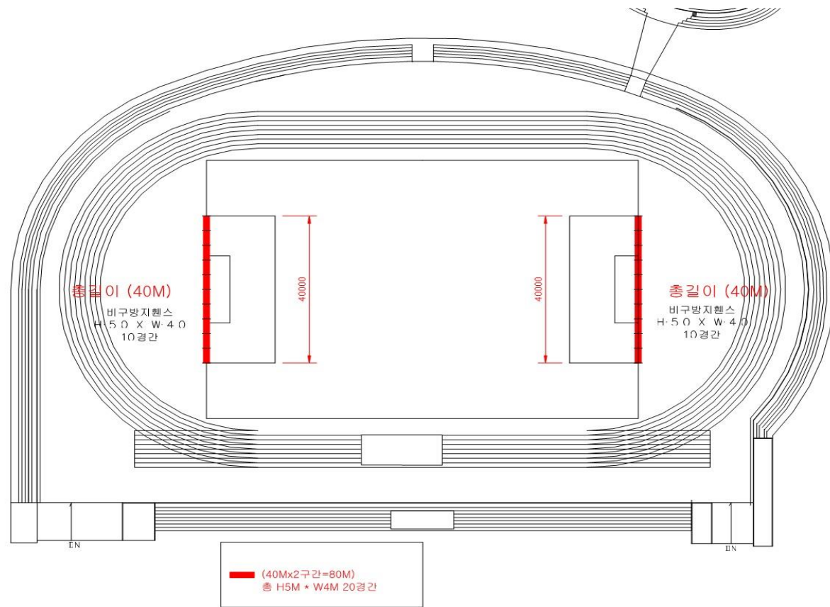
축구장 비구방지 휀스설치 평면도
